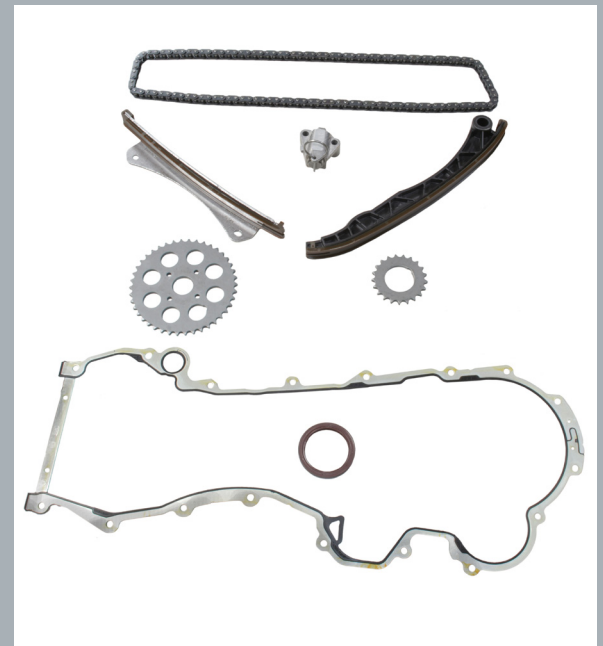
Bild 1: 3458010SD Vollsatz inkl. Dichtungen
