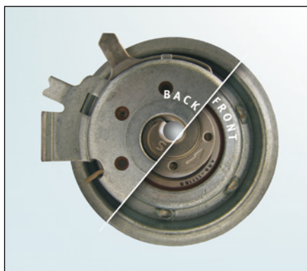
Bild 1: 531 0203 20 - bisherige Ausführung
