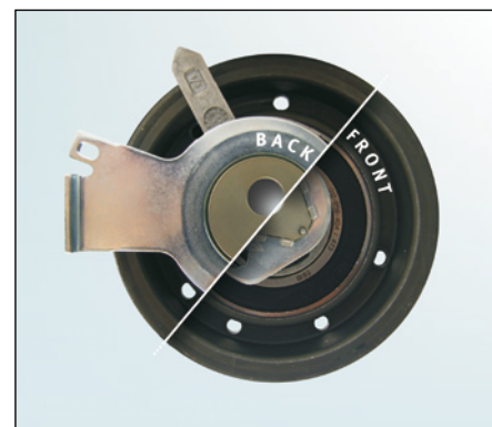
Bild 2: 531 0203 20 - neue Ausführung
