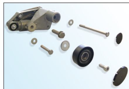
Bild 3: Lieferumfang 533 0097 10
