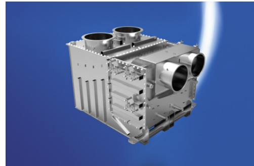
Abgasreinigungsanlage „mobiclean“ für eine 3.000-kW-Diesellokomotive zur Erfüllung der strengen zukünftigen Abgasnormen EU-Stufe IIIB und EU-Stufe IV.
