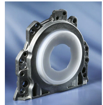
Integrierter PTFE-Radialwellendichtring mit Gehäuse und Montagehülse
